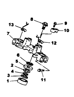
FIG.24 MESA DO GUIDÃO
