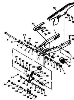
FIG.22 GARFO TRASEIRO
