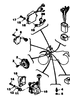
FIG.44 SISTEMA ELÉTRICO 2 P.51
