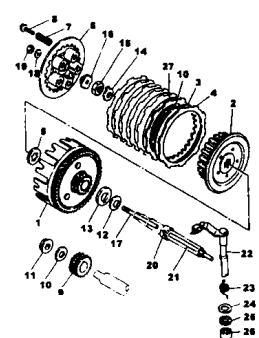
FIG.12 FRICÇÃO P.16
