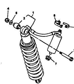
FIG.23 AMORTECEDOR TRASEIRO
